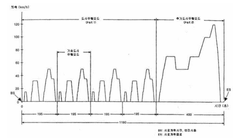
그림 2. 모드상세도
